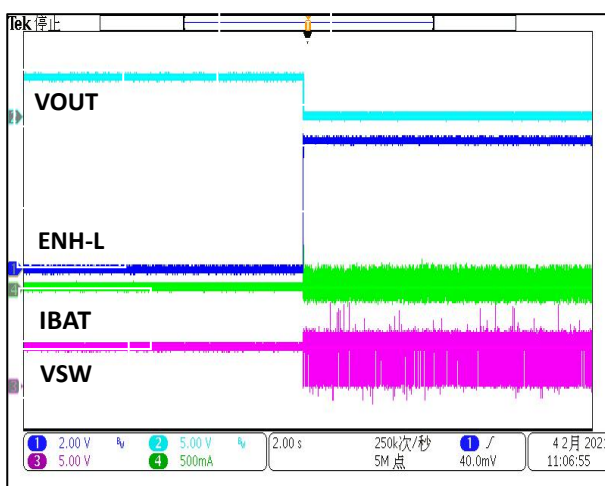
EN 高电平切换波形图
