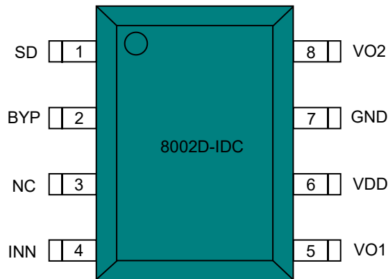
图2 8002D-IDC引脚定义图
