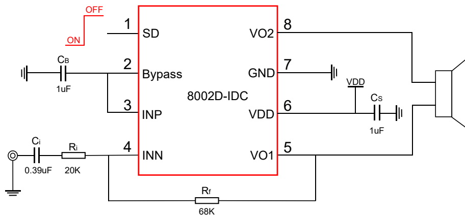
图3 8002D-IDC典型应用电路
