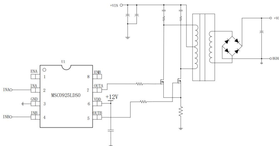
图1.1 MSC0925LDS0典型应用电路
