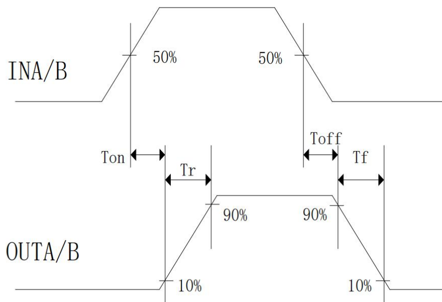
图1.3. 输出LO开关时间波形图
