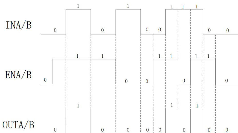
图1.4. 输入信号和输出信号逻辑功能图
