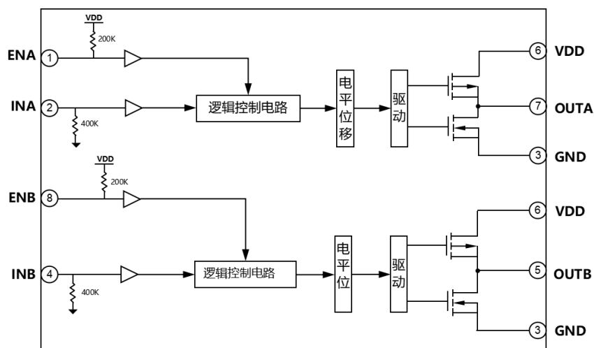
图1.2 MSC0925LDS0 内部电路图
