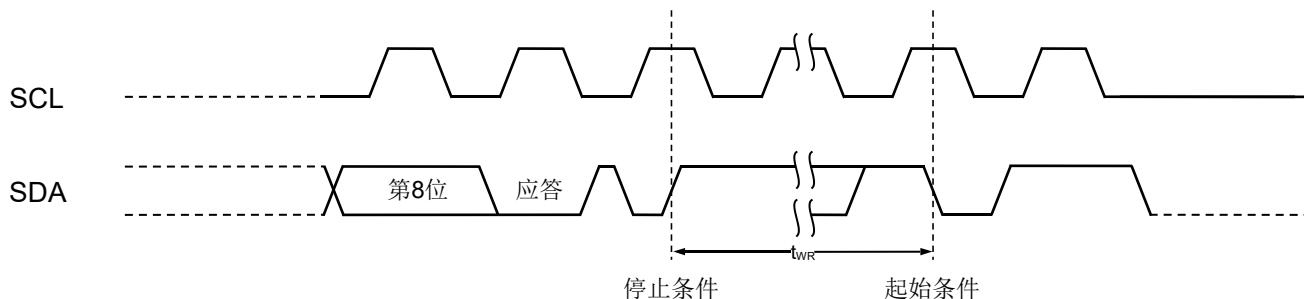
图5 总线时序
