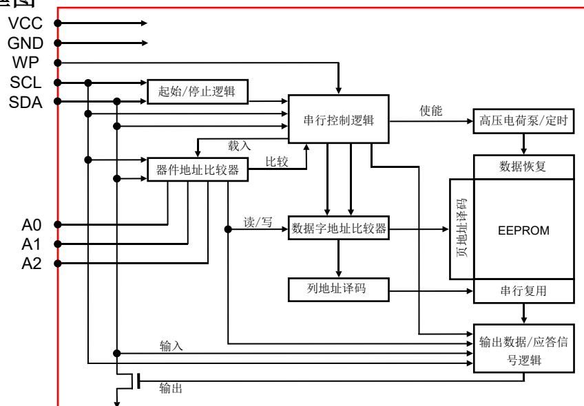
图1 AD24C02D内部原理框图
