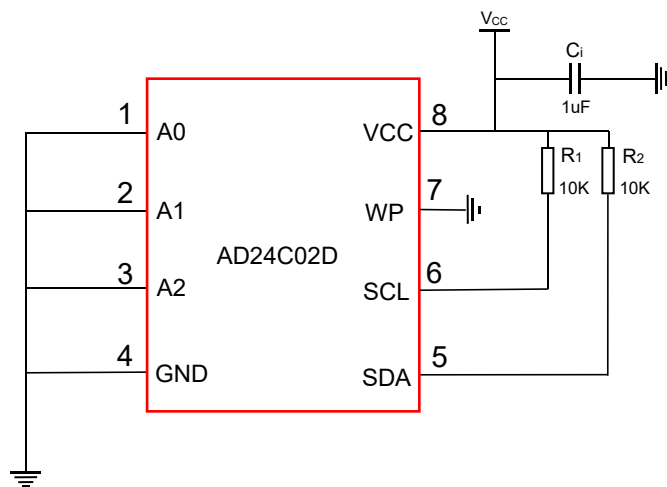
图3 AD24C02D典型应用电路
