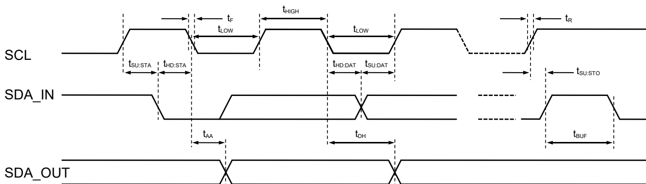
图5 总线时序
