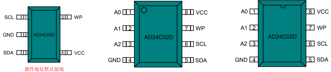
图2 AD24C02D引脚定义图
