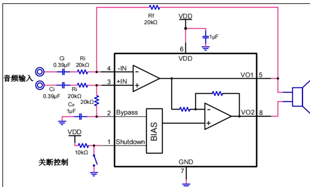
图 3. TPA6203 差分输入模式电路图
