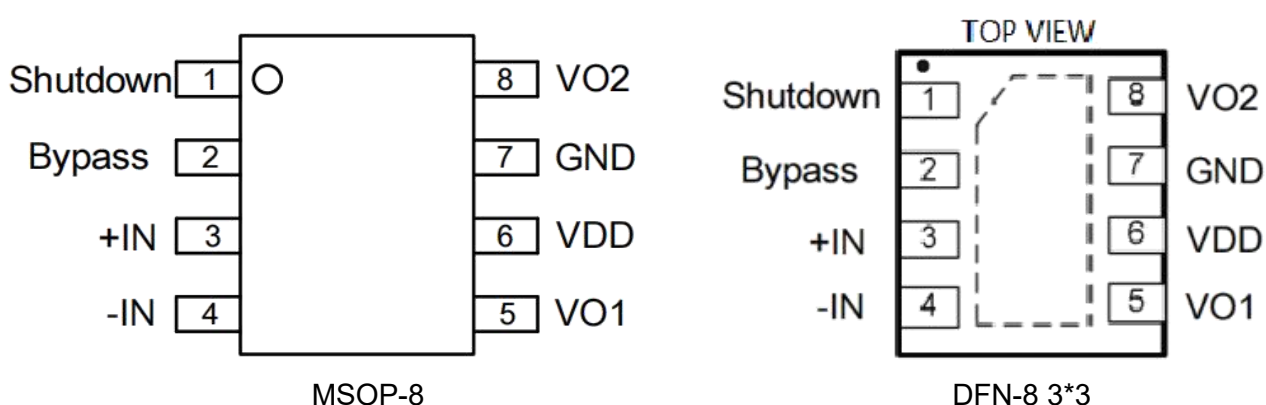
图 1. TPA6203 的管脚定义图
