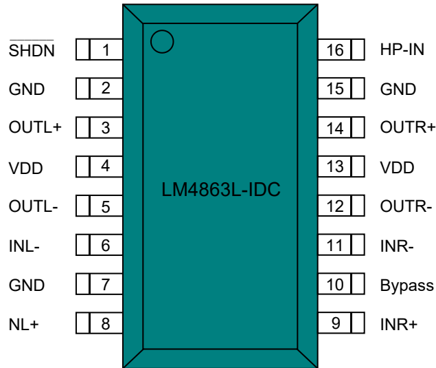
图2 LM4863L-IDC引脚定义图
