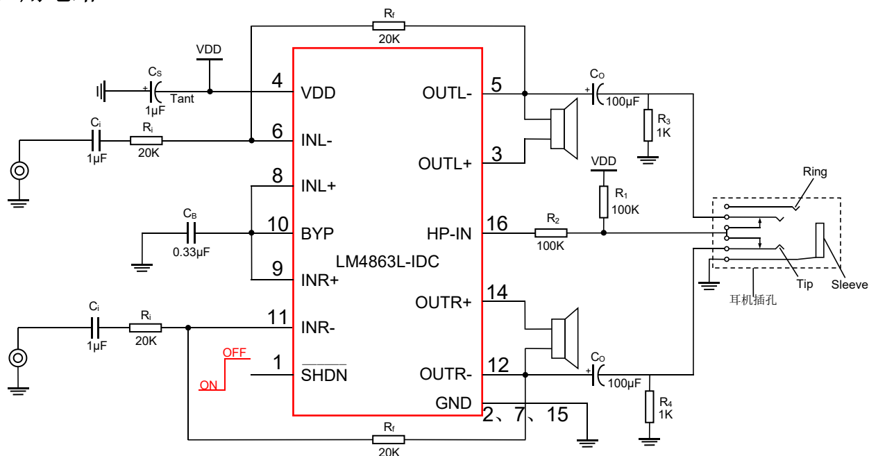
图3 LM4863L-IDC典型应用电路
