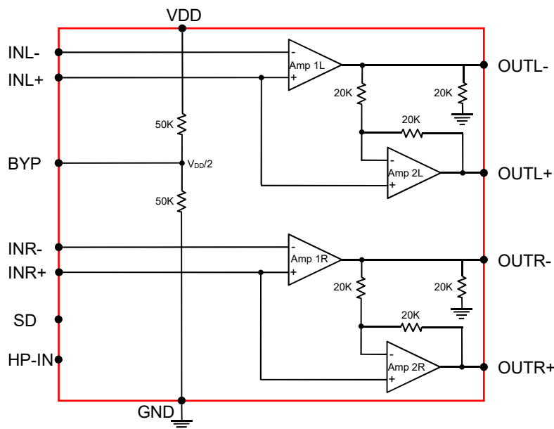
图1 LM4863L-IDC内部原理框图
