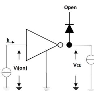
图 4 V I(on) 测试电路
