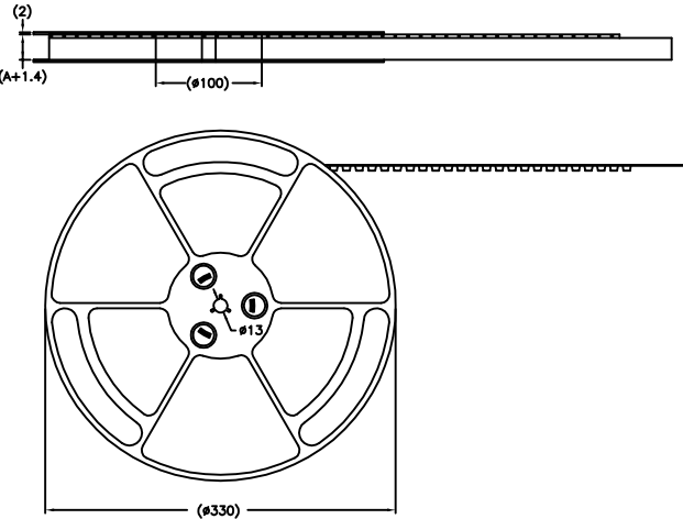
REEL Dim
