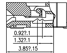
CABLE INSERT DIM. SCALE 2:1
