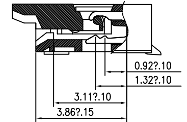
CABLE INSERT DIM. SCALE 2:1
