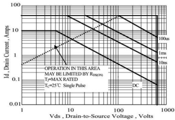
图 6(T0-220) 最大安全工作区曲线 Fig6 Maximum Safe OperatingArea
