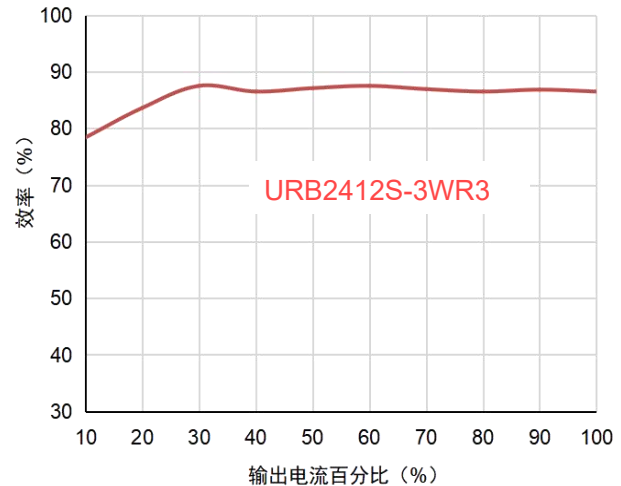
效率VS输出负载（标称输入）
