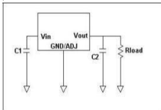
图 1 1117 固定电压版本应用电路
