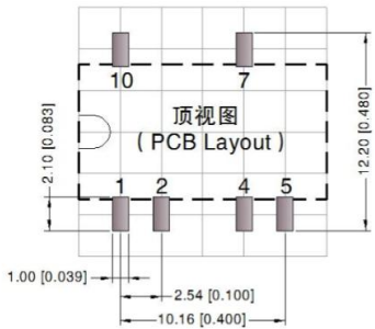
注：栅格距离为2.54*2.54mm
