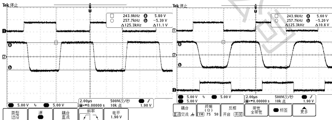
图 1.SP3232EEY-L-HX 在速率为 250kbps 时驱动器输入与输出波形 (无负载)
