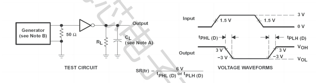
图 3. 驱动器传输转换速率测试电路
