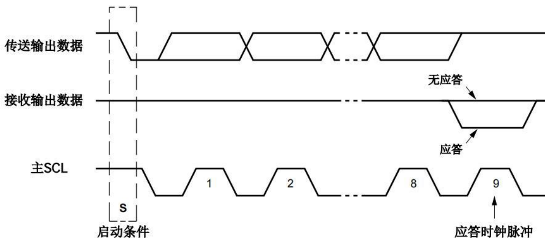
图6、I 2 C总线标志位
