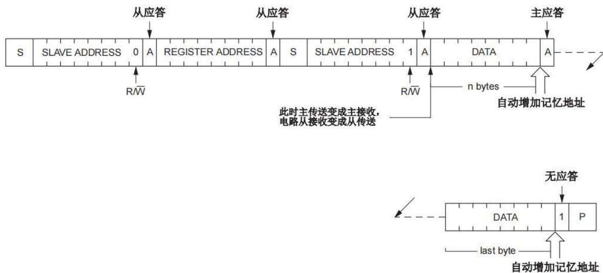
图9、设置字地址后主设备读数据（写字地址：读数据）
