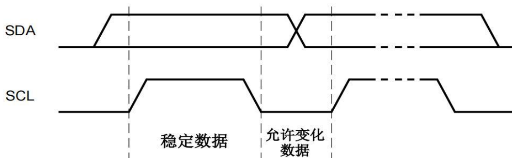
图5、I 2 C总线位传送
