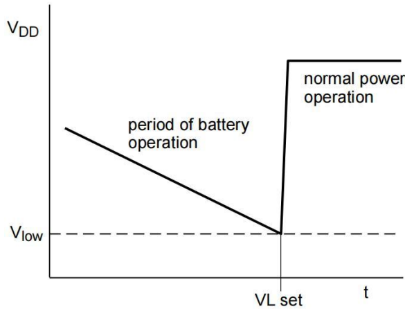
图1、低电压检测器
