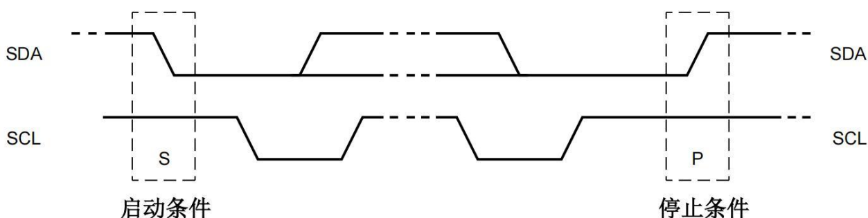
图4、I 2 C总线启动和停止条件
