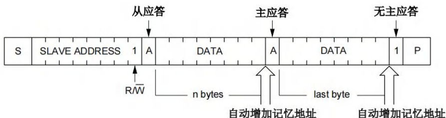
图10、主设备读从设备第一个字节数据后的数据（读模式）
