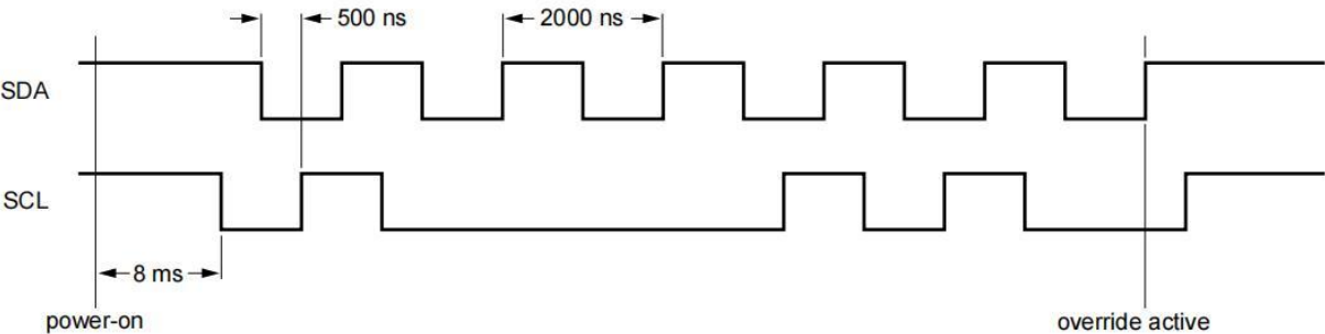
图2、POR失败时序图
