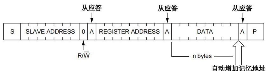
图8、主传送器到从接收器（写模式）
