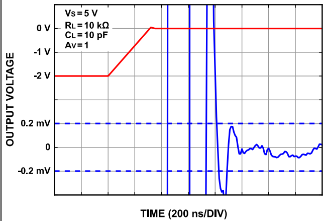
Figure 24. Rising Edge Settling
