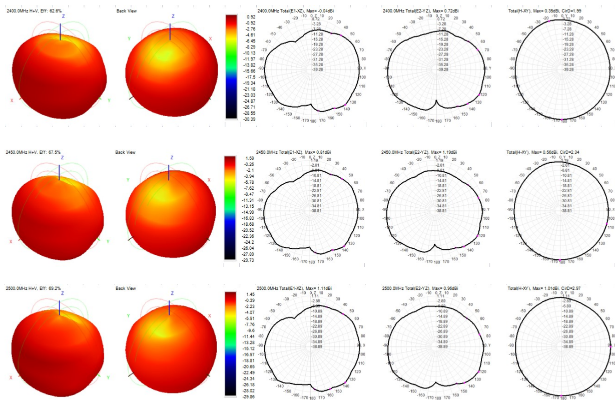
图 10 天线场型图
