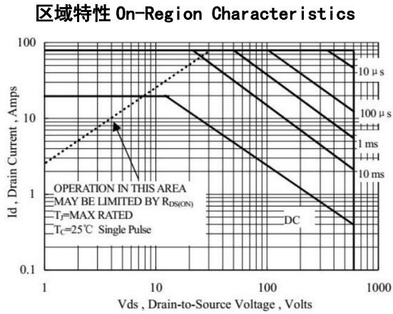
图 6(T0-220) 最大安全工作区曲线 Fig6 Maximum Safe OperatingArea
