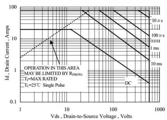
图 9(T0-247) 最大安全工作区曲线 Fig7 Maximum Safe OperatingArea
