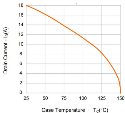
图 5 最大漏极电流与壳温曲线 Fig5 Maximum Drain Current Vs. Case Temperature
