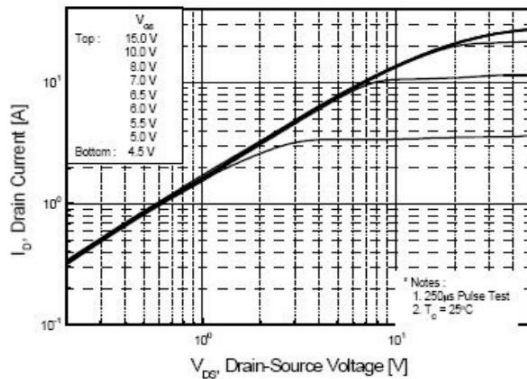
图 1 输出特性曲线, T_c=25^\circ\text{C}
