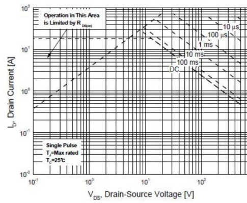
图 7(T0-220FP)最大安全工作区曲线 Fig7 Maximum Safe OperatingArea
