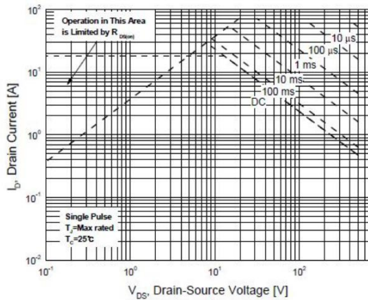
图 8(T0-262&263)最大安全工作区曲线 Fig8 Maximum Safe OperatingArea
