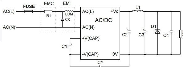
推荐电路 2
