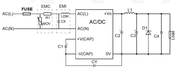
推荐电路 3
