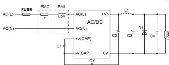
推荐电路 1
