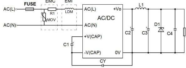
推荐电路 4
