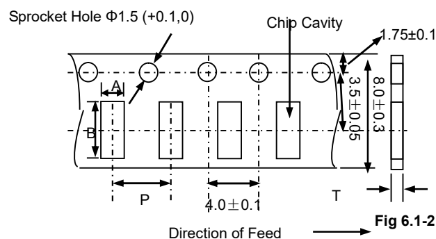
Type A B P T max H 3216[1206] 1.9±0.2 3.5±0.2 4.0±0.1 1.1 10
