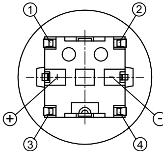
开关底部图
