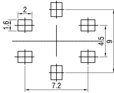
P. C. B. LAYOUT
