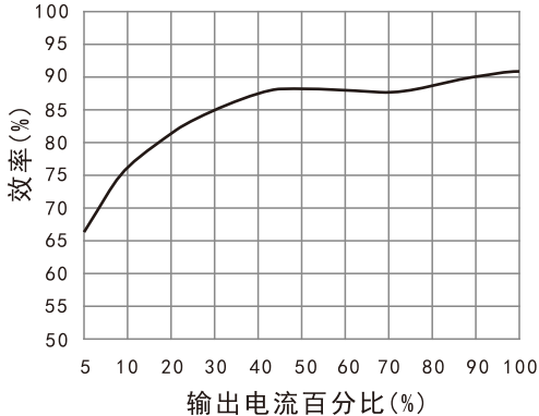
效率Vs输出负载( V_{in}=48\text{V} ) URF4815P-6WR3
