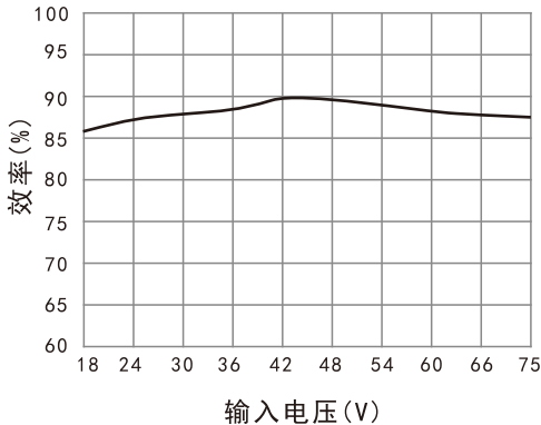
效率Vs输入电压(满载) URF4815P-6WR3
