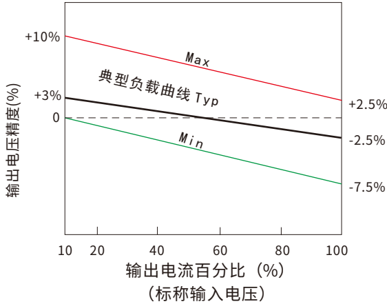
误差包络曲线图 5Vdc输出
