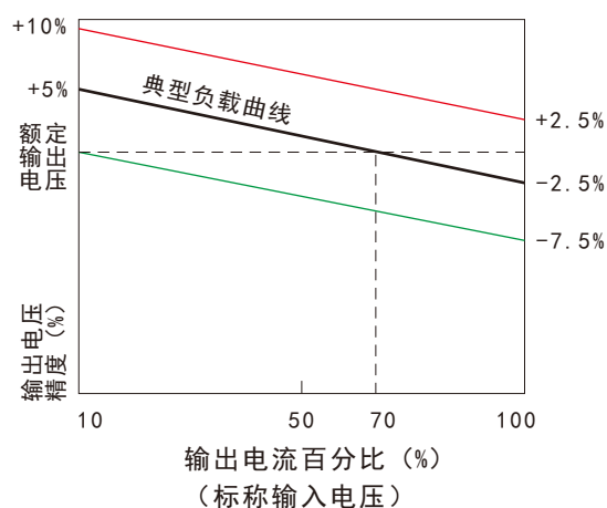
误差包络曲线图
