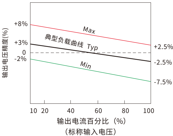
误差包络曲线图 其它输出
