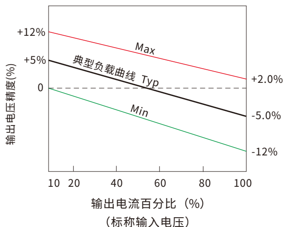
误差包络曲线图 3.3Vdc输出
