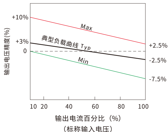
误差包络曲线图 5Vdc输出
