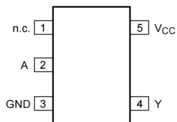
SOT23-5 / SOT353
