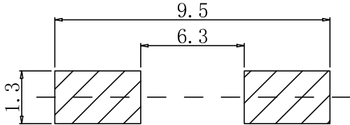
线 路 板 图 PCB Diagram
