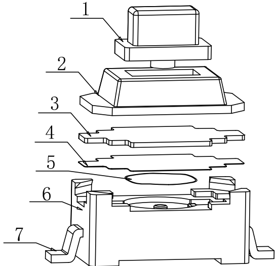
分解图
