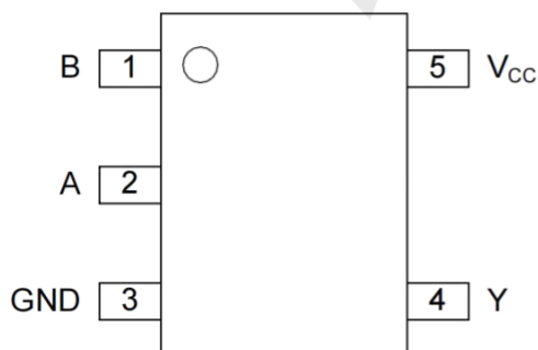
SOT23-5 / SOT353
