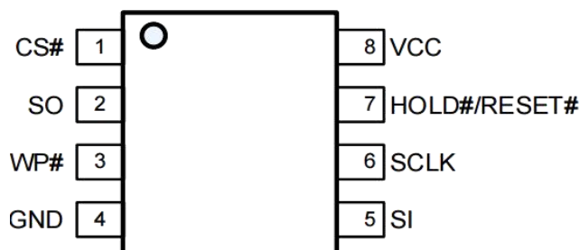
SOP-8(150MIL/208MIL)
