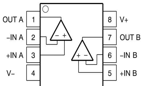
TSV912 SOP8/MSOP8/TSSOP8 Pin Diagram
