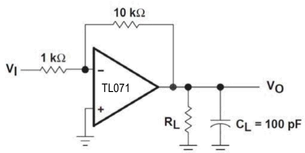
图 2. 10 倍增益电路
