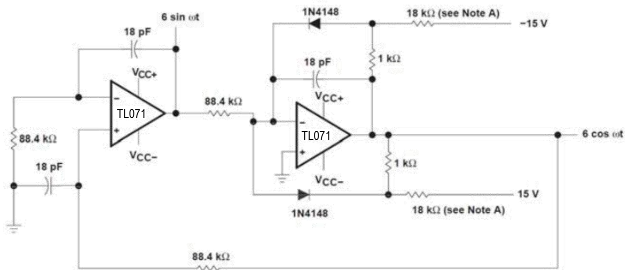
图 3. 100KHz 振荡器
