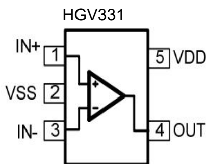
SOT-23-5/SC70-5
