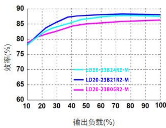
效率 VS 输出负载曲线图（Vin=230VAC）
