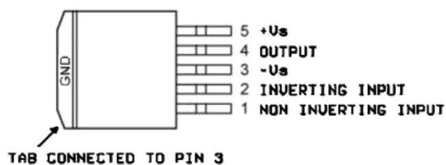
TO-263-5
