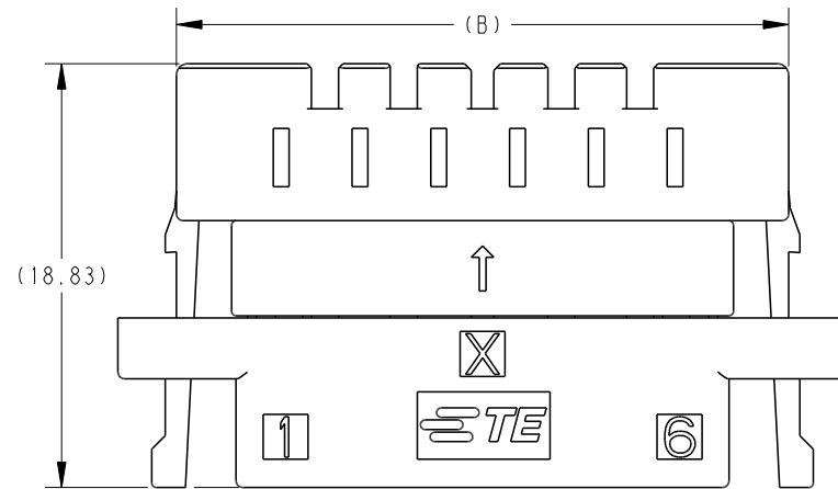
P/N: 1-2473514-6 (6POS:X-KEY)
