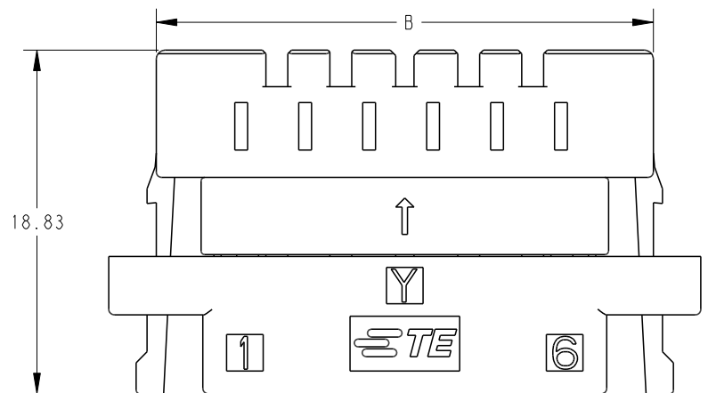
P/N: 2-2473514-6 (6POS:Y-KEY)
