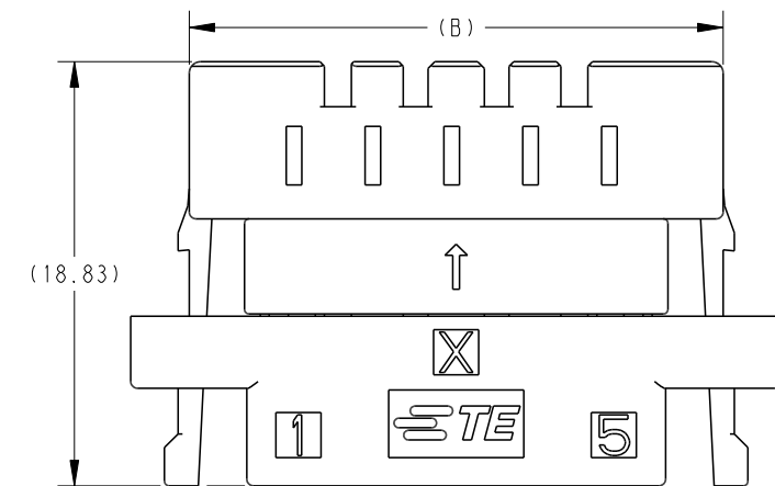
P/N: 1-2473514-5 (5POS:X-KEY)
