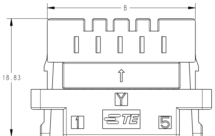
P/N: 2-2473514-5 (5POS:Y-KEY)
