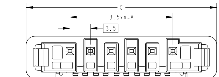
P/N: 1-2473514-6 (6POS:X-KEY)
