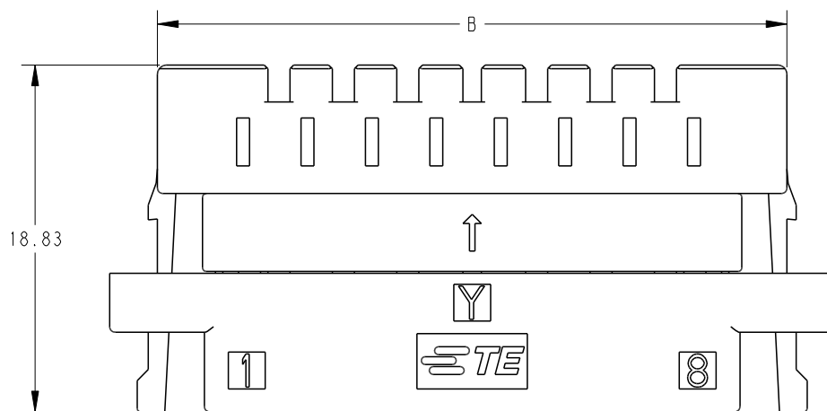
P/N: 2-2473514-8 (8POS:Y-KEY)
