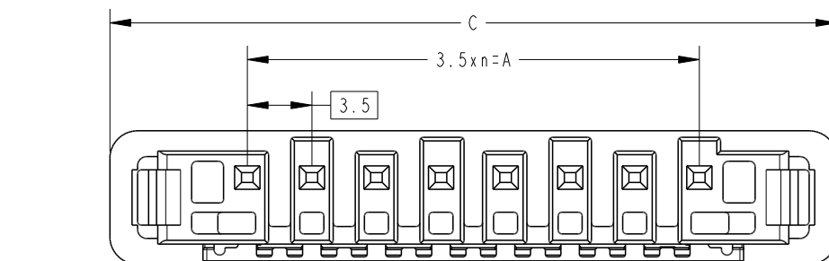
P/N: 1-2473514-8 (8POS:X-KEY)
