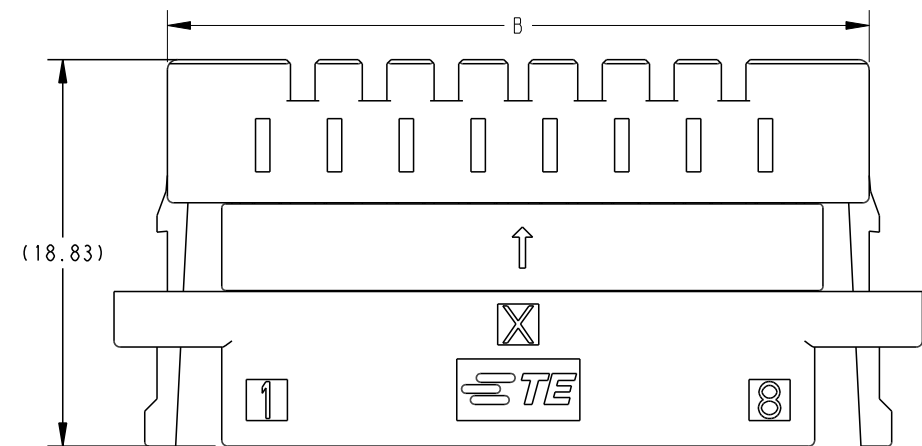
P/N: 1-2473514-8 (8POS:X-KEY)
