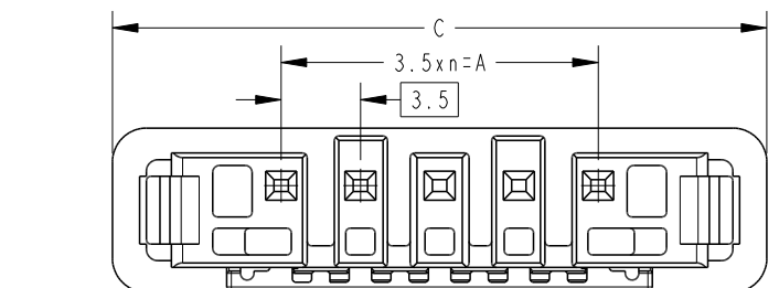
P/N: 1-2473514-5 (5POS:X-KEY)
