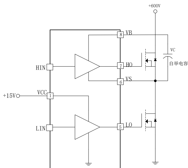
图 8-3. EG2106S 自举电路结构
