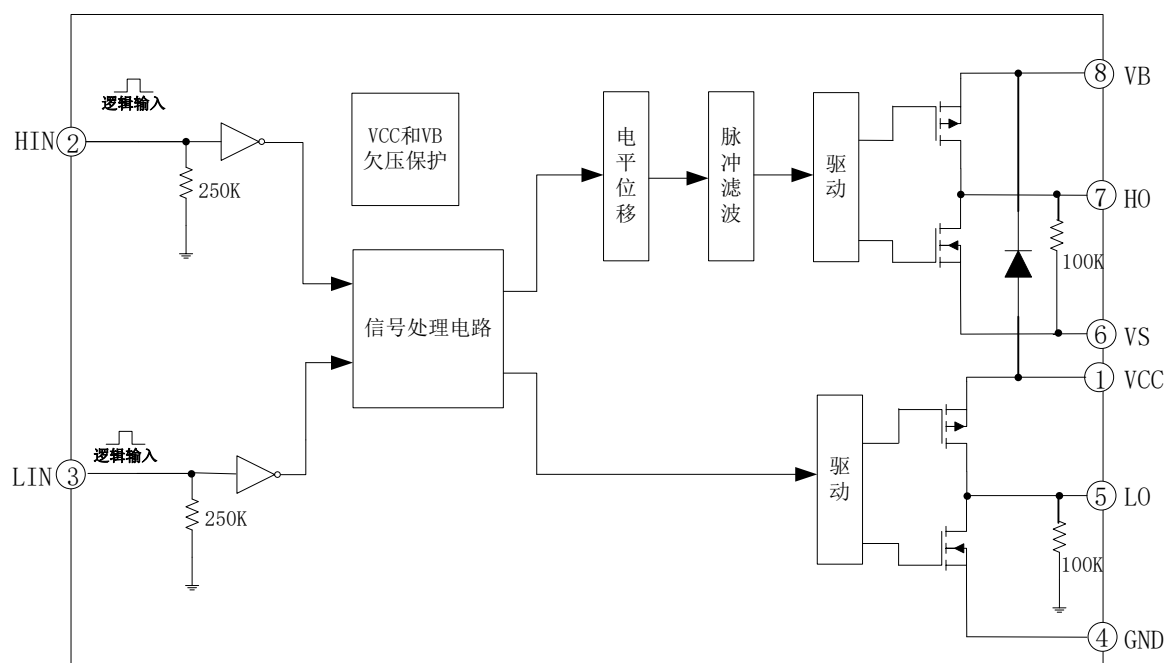
图 5-1. EG2106S 内部电路图
