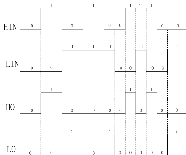
图8-2. 输入信号和输出信号逻辑功能图
