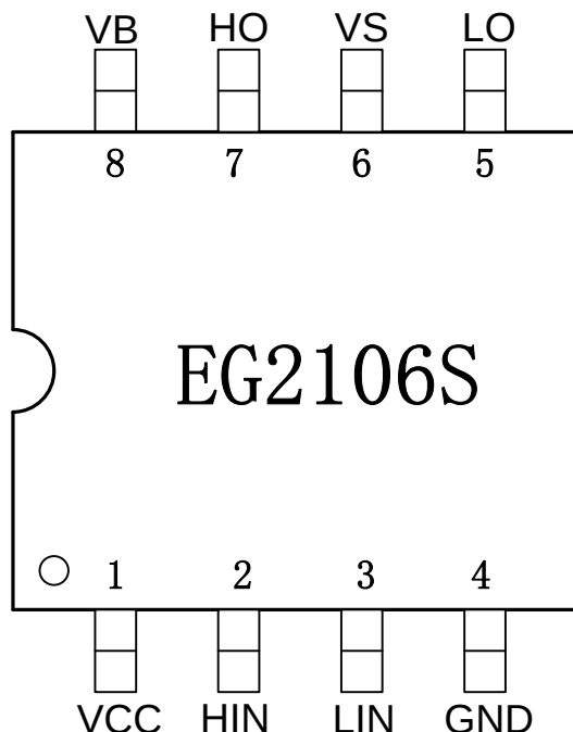
图 4-1. EG2106S 管脚定义
