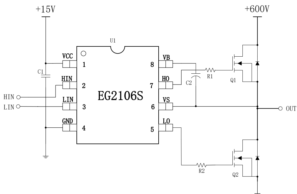
图 6-1. EG2106S 典型应用电路图
