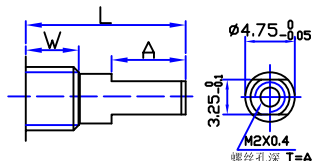
SE Shaft Style
