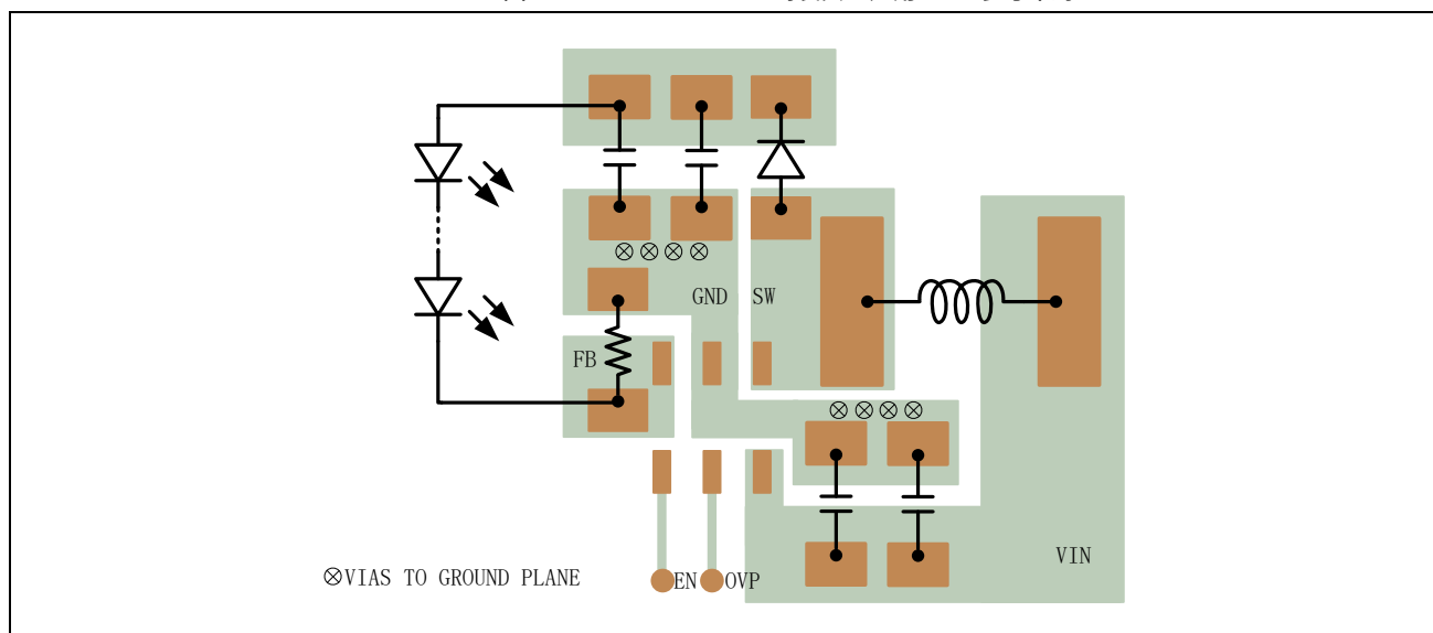
图 15.2 Boost 型 SOT23-6 封装典型应用 PCB 参考布局
