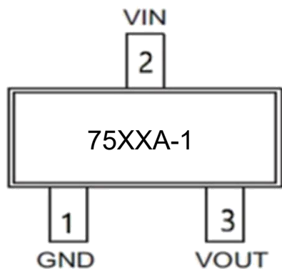
SOT-23-3
