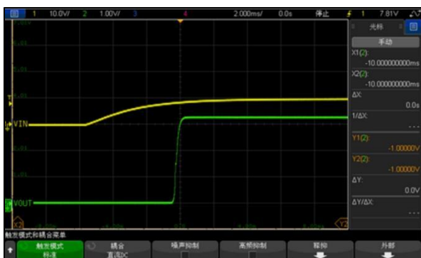
Vin=10V,Iout=0mA,Cout=0.1uF
