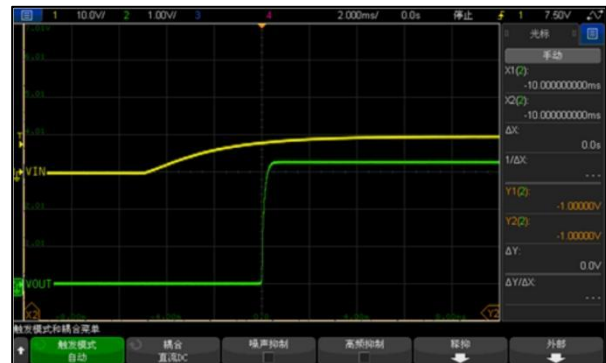
Vin=10V,Iout=0mA,Cout=10uF
