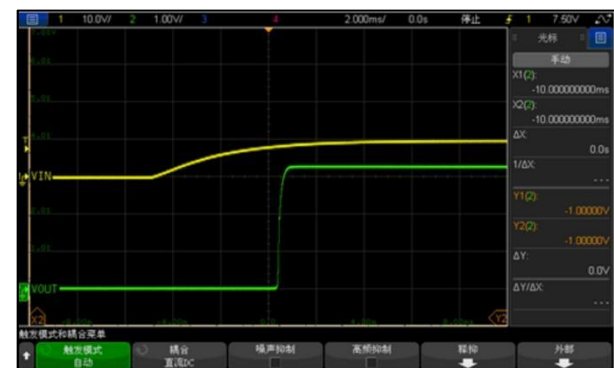
Vin=10V,Iout=30mA,Cout=10uF
