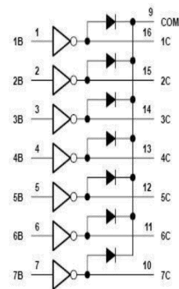
ULN2003AL 逻辑
