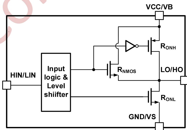
图 10-2 NSG3027 输出级示意图
