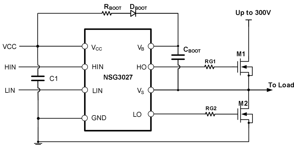
图 11-1 典型应用电路图
