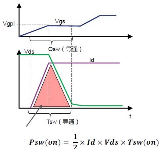
图 11-3 阻性负载条件下的 MOS 开关损耗
