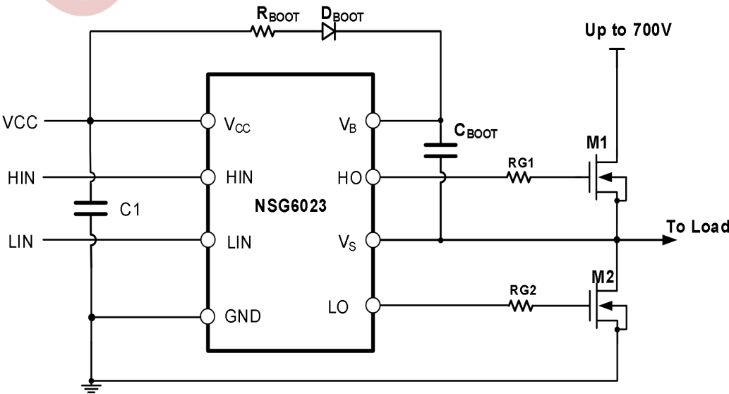
图 11-1 典型应用电路图
