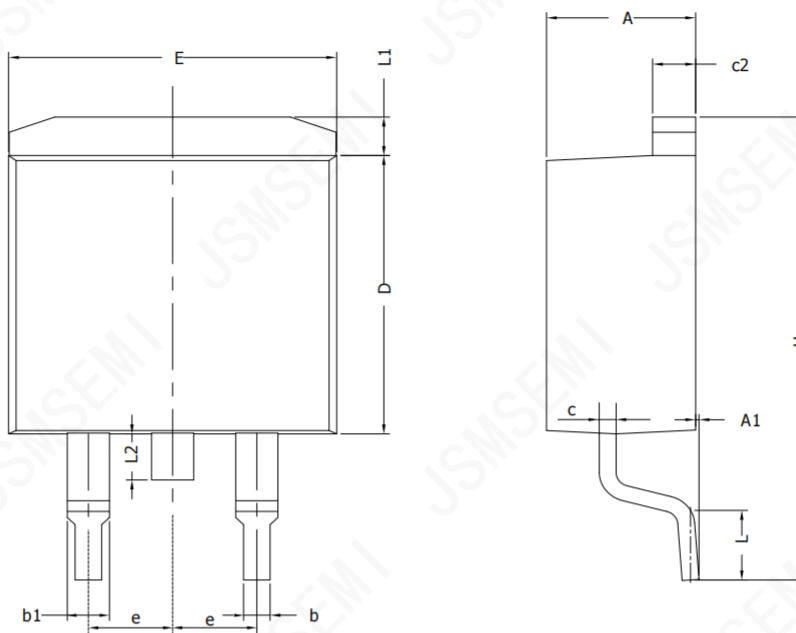
TO-263-2
