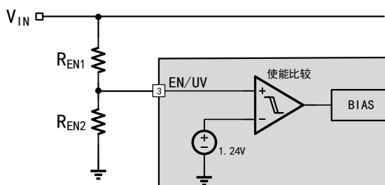
图7.3 IBSP3030UVLO典型应用
