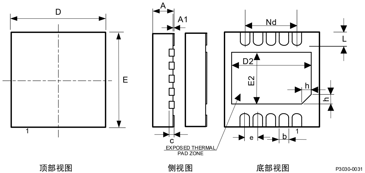
图11.1 IBSP3030DFN10封装
