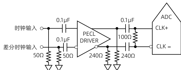
图 16 差分 PECL 采样时钟
