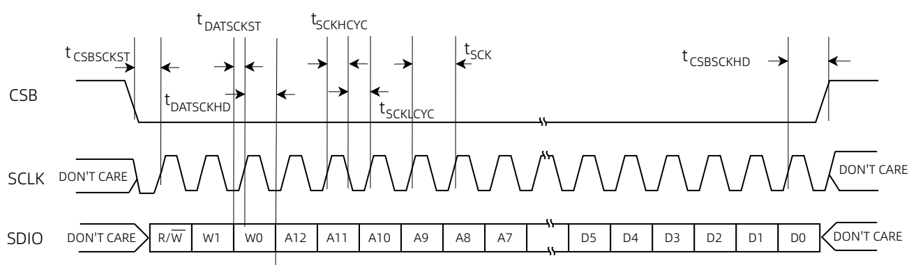
图 17 SPI 接口时序图
