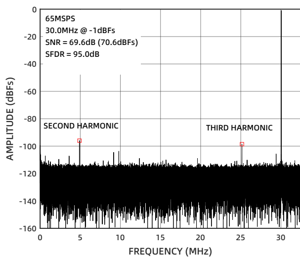
图 4 单音 FFT ( f_{IN} = 30\text{MHz} )
