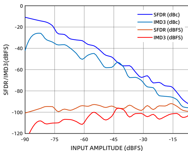
图 8 双音 SFDR/IMD3 随输入幅度的变化 ( f_{IN} = 30\text{MHz} )
