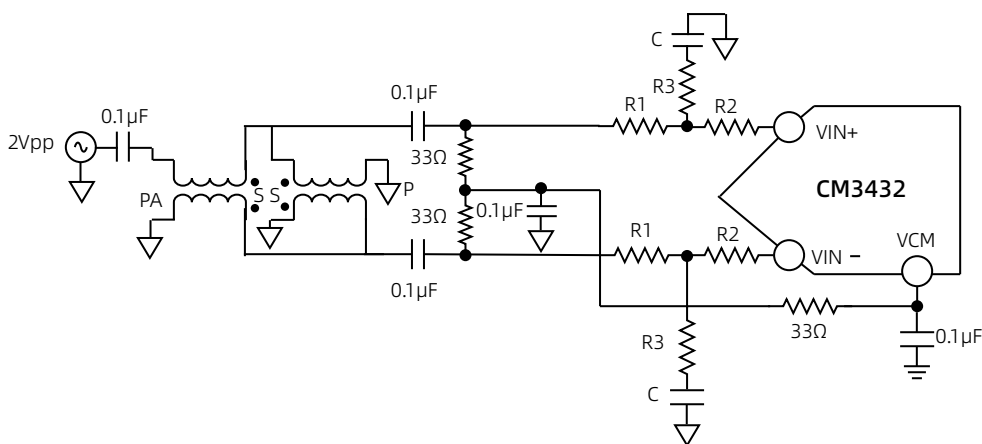
图 13 差分双巴比伦输入配置
