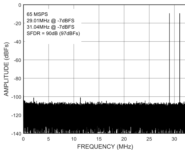
图 5 双音 FFT ( f_{IN} = 30\text{MHz} )
