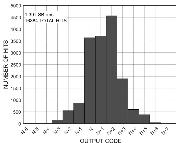
图 9 零输入直方图
