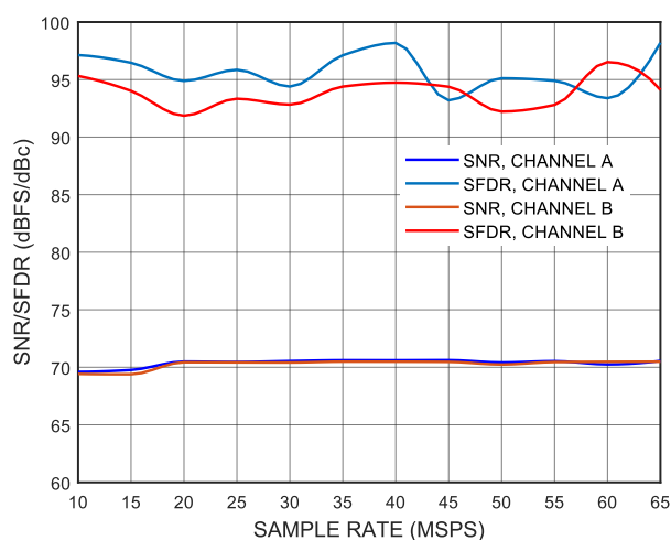
图 7 单音 SNR/SFDR 随采样率的变化 ( f_{IN} = 30\text{MHz} )
