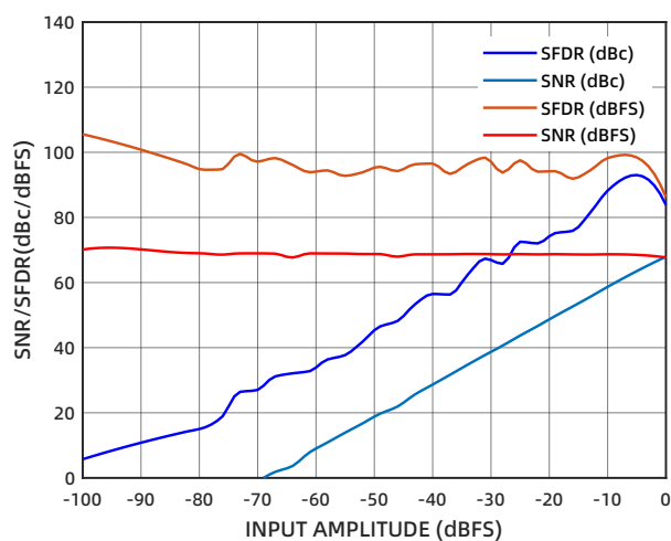
图 6 单音 SNR/SFDR 随输入幅度的变化 ( f_{IN} = 30\text{MHz} )
