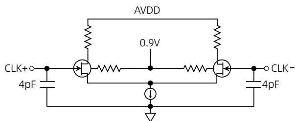
图 14 简易等效时钟输入电路
