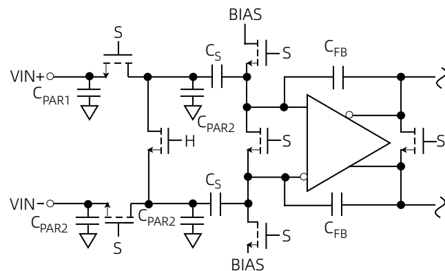
图 11 开关电容输入
