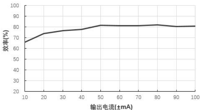
效率Vs输出电流( V_{in}=12V )@A1205LS-1WN
