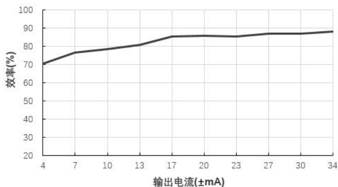
效率Vs输出电流( V_{in}=5V )@A0515LS-1WN
