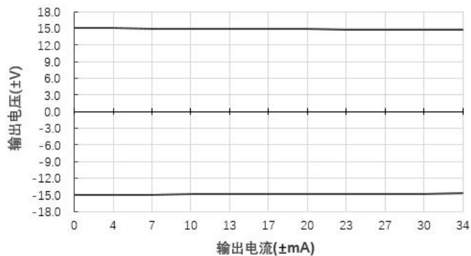
输出电压Vs输出电流( V_{in}=24V )@A2415LS-1WN
