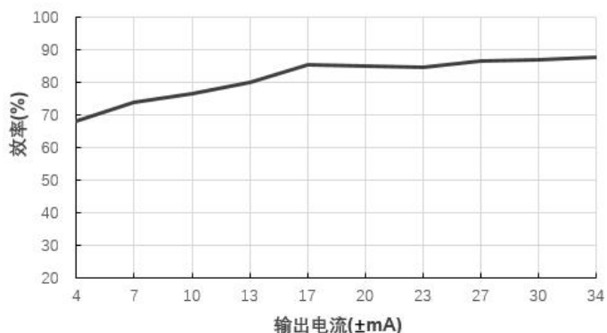
效率Vs输出电流( V_{in}=12V )@A1215LS-1WN
