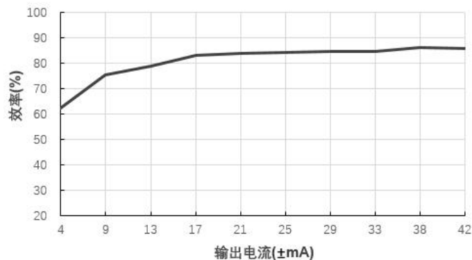
效率Vs输出电流( V_{in}=12V )@A1212LS-1WN
