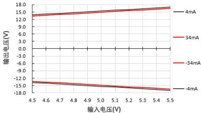
输出电压Vs输入电压@A0515LS-1WN
