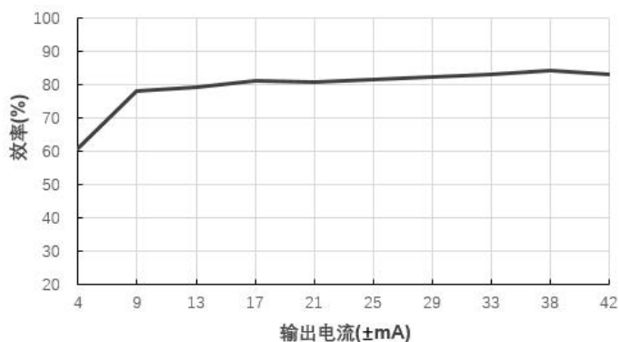
效率Vs输出电流( V_{in}=5V )@A0512LS-1WN
