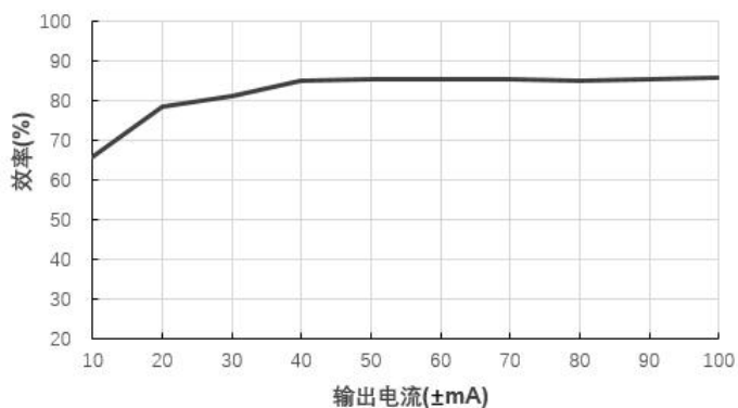
效率Vs输出电流( V_{in}=5V )@A0505LS-1WN
